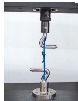
Test d'arrachement suivant la norme Européenne
