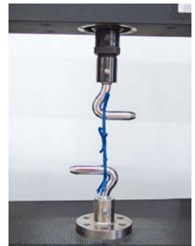
Test d'arrachement de la norme Européenne.
