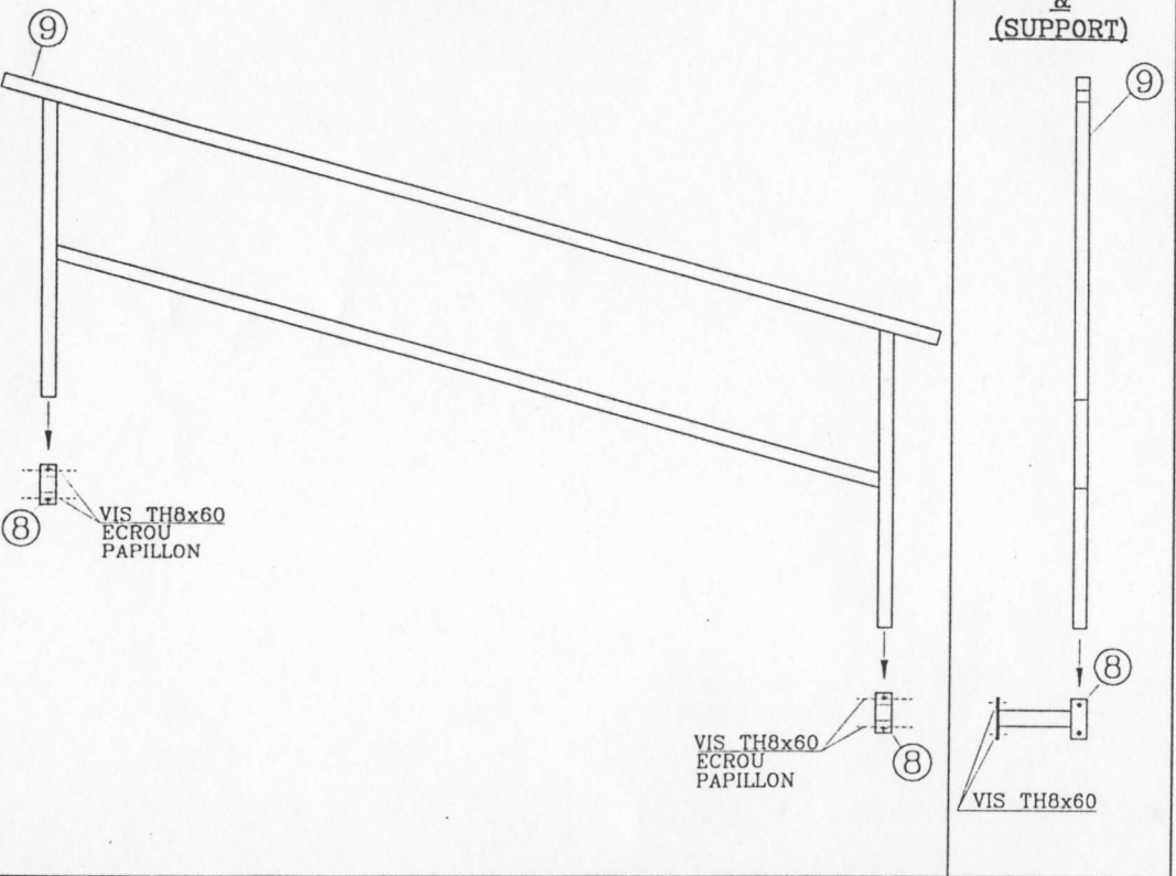
VUE DE PROFIL (GARDE FOU & SUPPORT)
