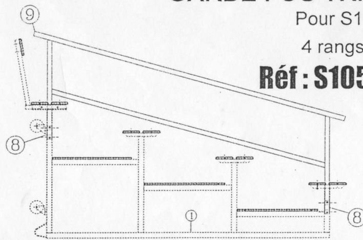
VUE DE FACE "A" (GARDE FOU) & (SUPPORT)
