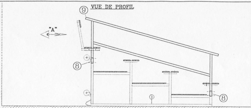
VUE DE PROFIL (GARDE FOU & SUPPORT)
