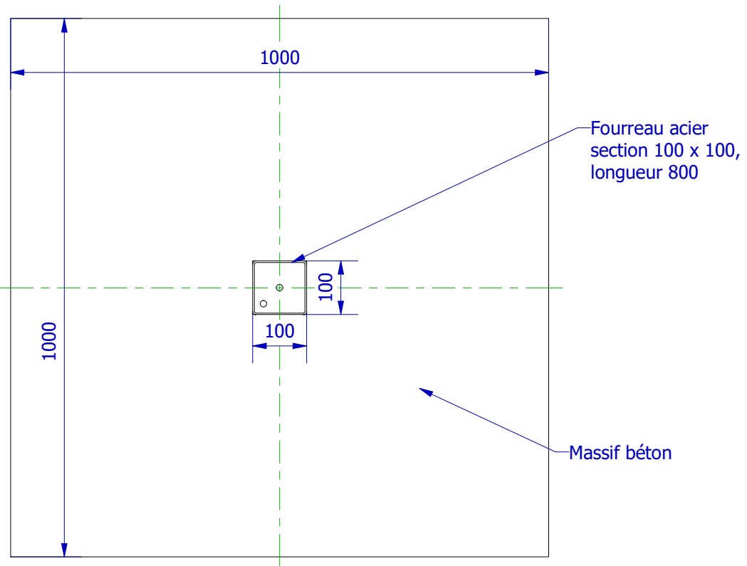
A ( 1 : 10 )
