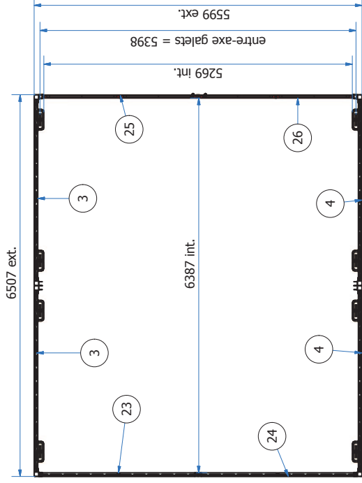
A-A ( 1 : 45 )
