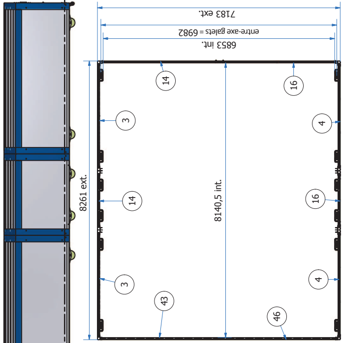
A-A ( 1 : 55 )
