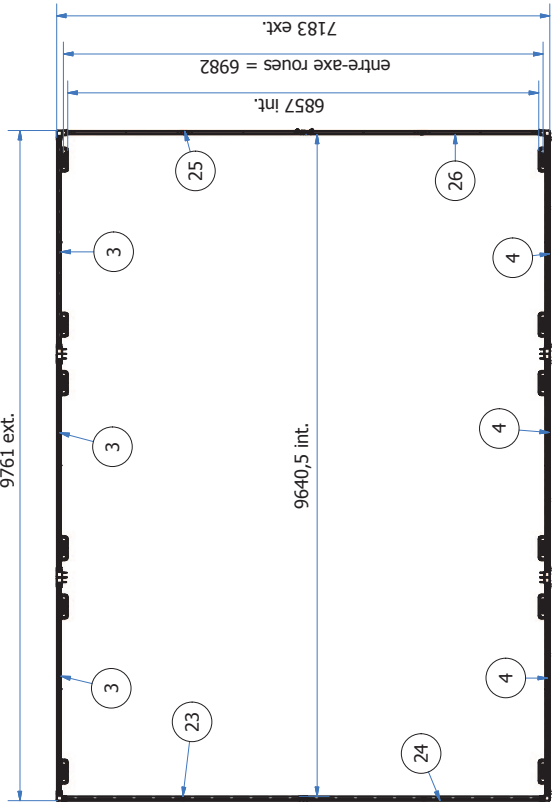
A-A ( 1 : 55 )
